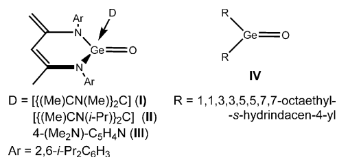
Figure 1. Structure of germanones I–IV . The donor ligand (D) corresponds to ligand \text{L}' .
